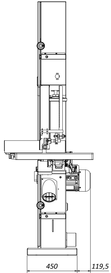
Näkymä sivulta:
